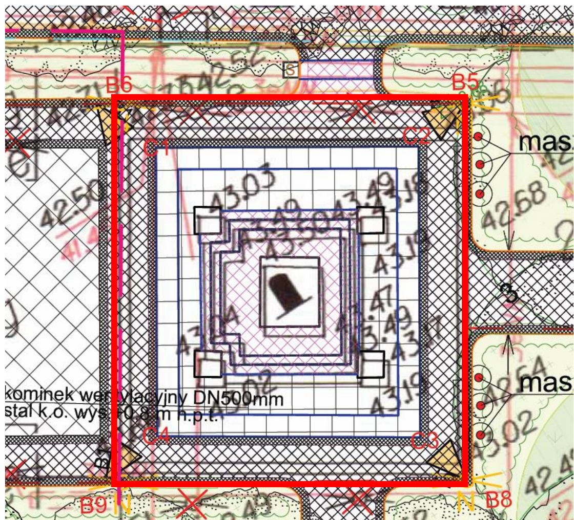
Zaznaczony fragment pomnika – kwadrat o wymianak ok. 14 m x ok. 14 m
